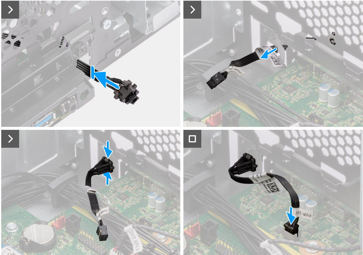
Obrázek 69. Montáž vypínače
