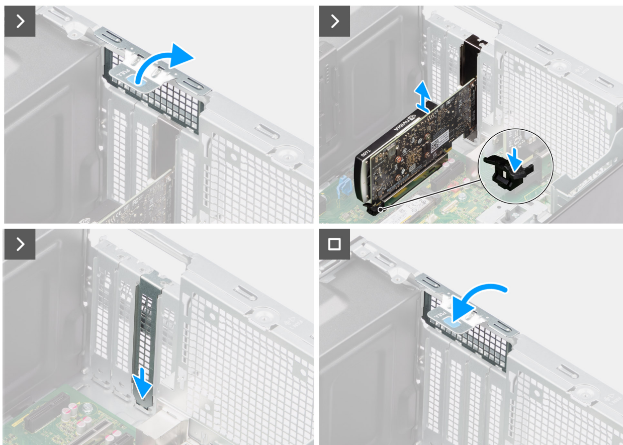
Obrázek 38. Demontáž grafické karty
