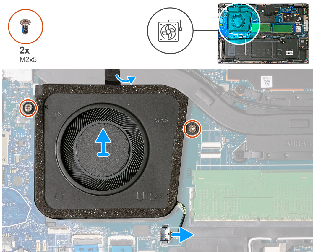
Obrázek 24. Demontáž ventilátoru
