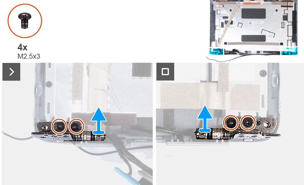
Obrázek 60. Demontáž pantů displeje
