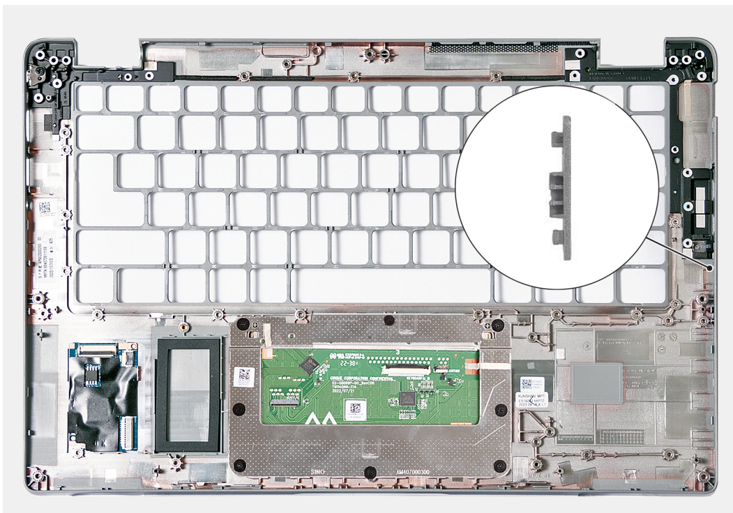
Obrázek 83. Demontáž sestavy opěrky pro dlaň
