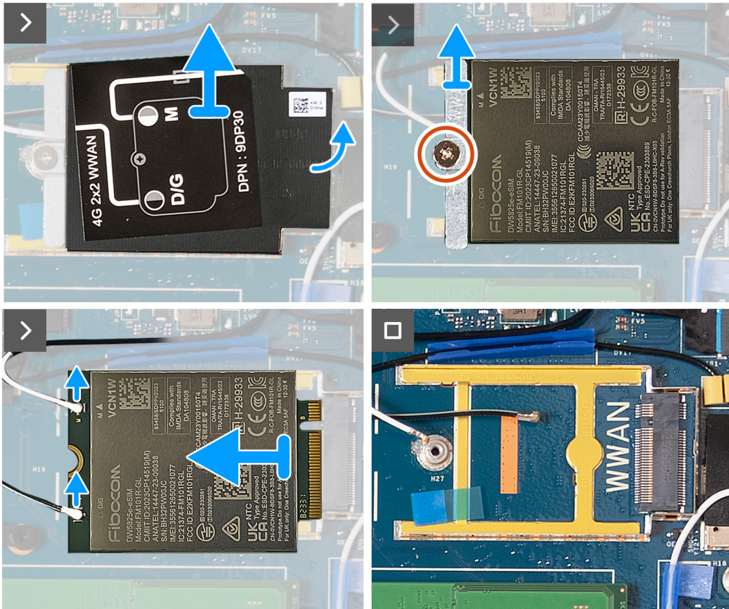
Obrázek 20. Demontáž karty WWAN – pro počítače dodávané s kartou 4G
