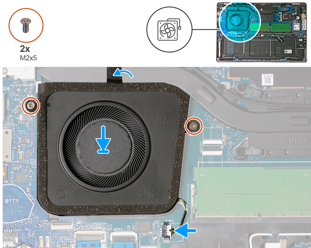
Obrázek 25. Montáž ventilátoru
