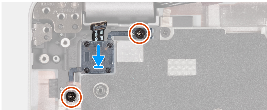
Obrázek 78. Montáž desky vypínače
