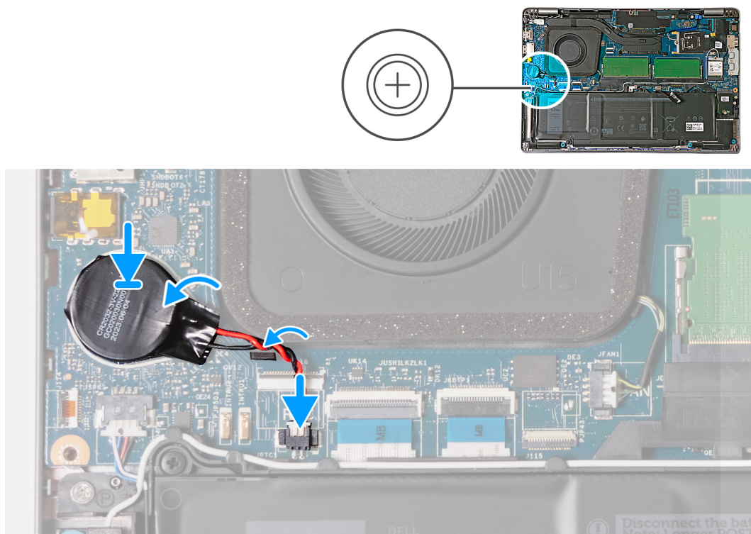
Obrázek 29. Montáž knoflíkové baterie
