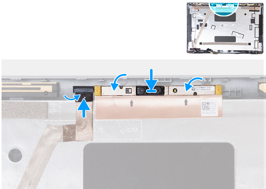
Obrázek 59. Montáž modulu kamery
