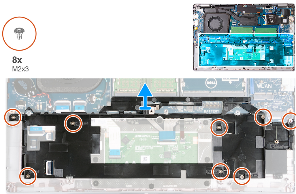
Obrázek 41. Demontáž vnitřního rámu sestavy
