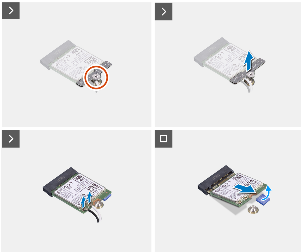
Obrázek 18. Demontáž bezdrátové karty
