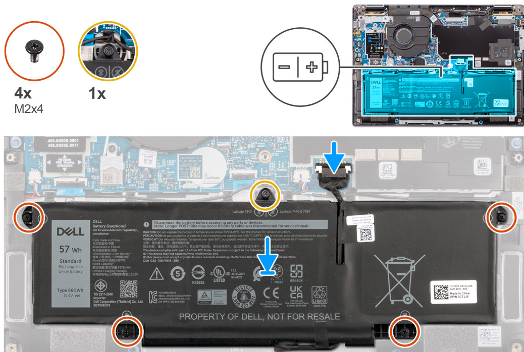
Obrázek 32. Montáž 4čládkové baterie
