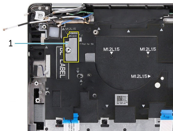
Obrázek 65. Podpůrná deska klávesnice pro 5G WWAN
