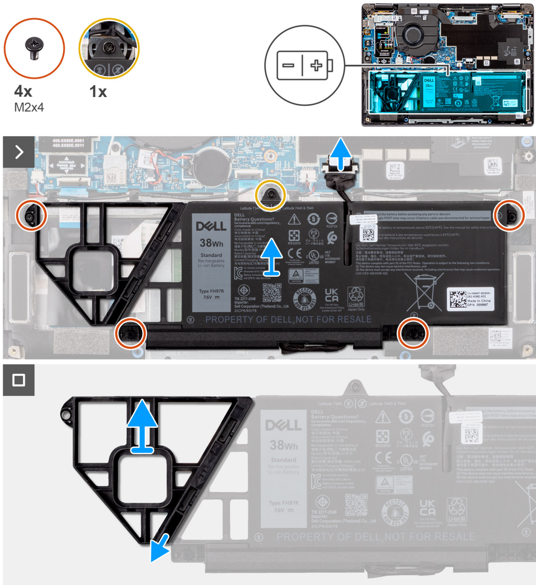
Obrázek 29. Demontáž 3článkové baterie
