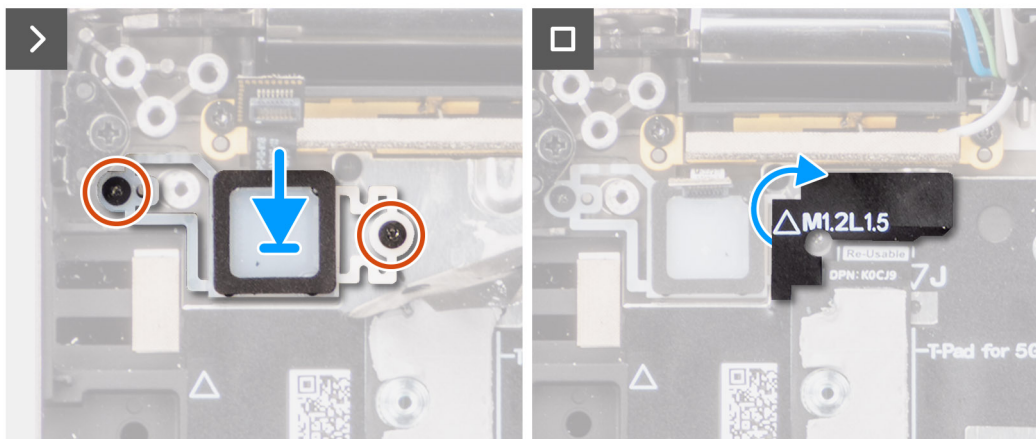
Obrázek 61. Montáž vypínače
