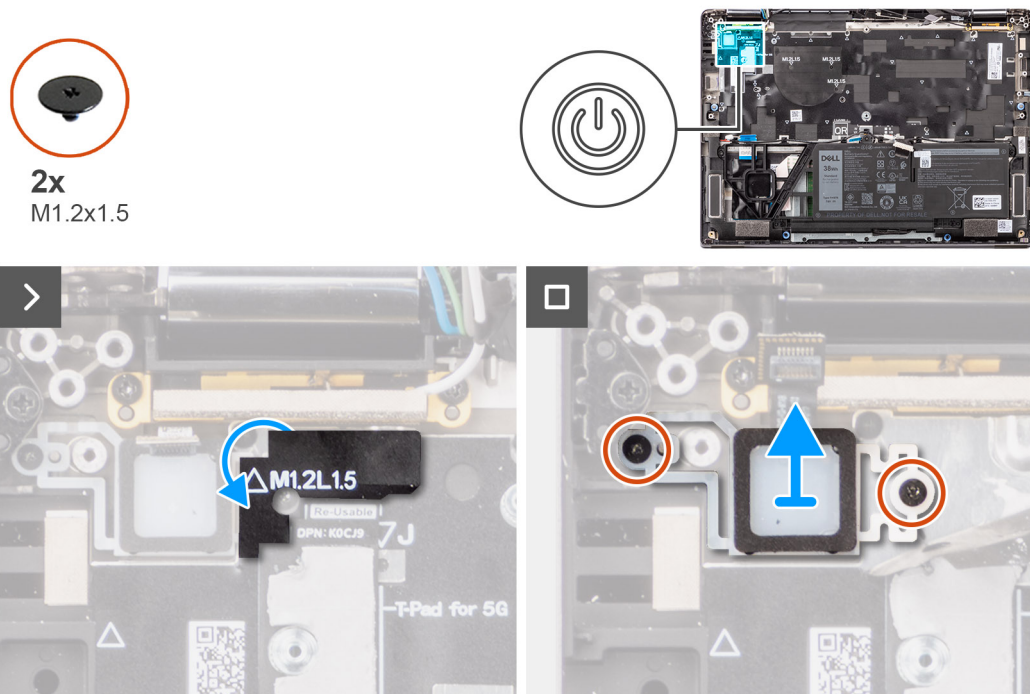
Obrázek 60. Demontáž vypínače
