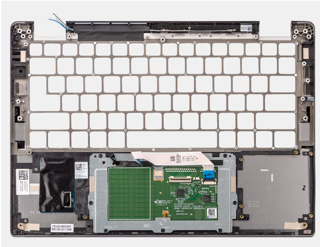
Obrázek 69. Montáž sestavy opěrky pro dlaň
