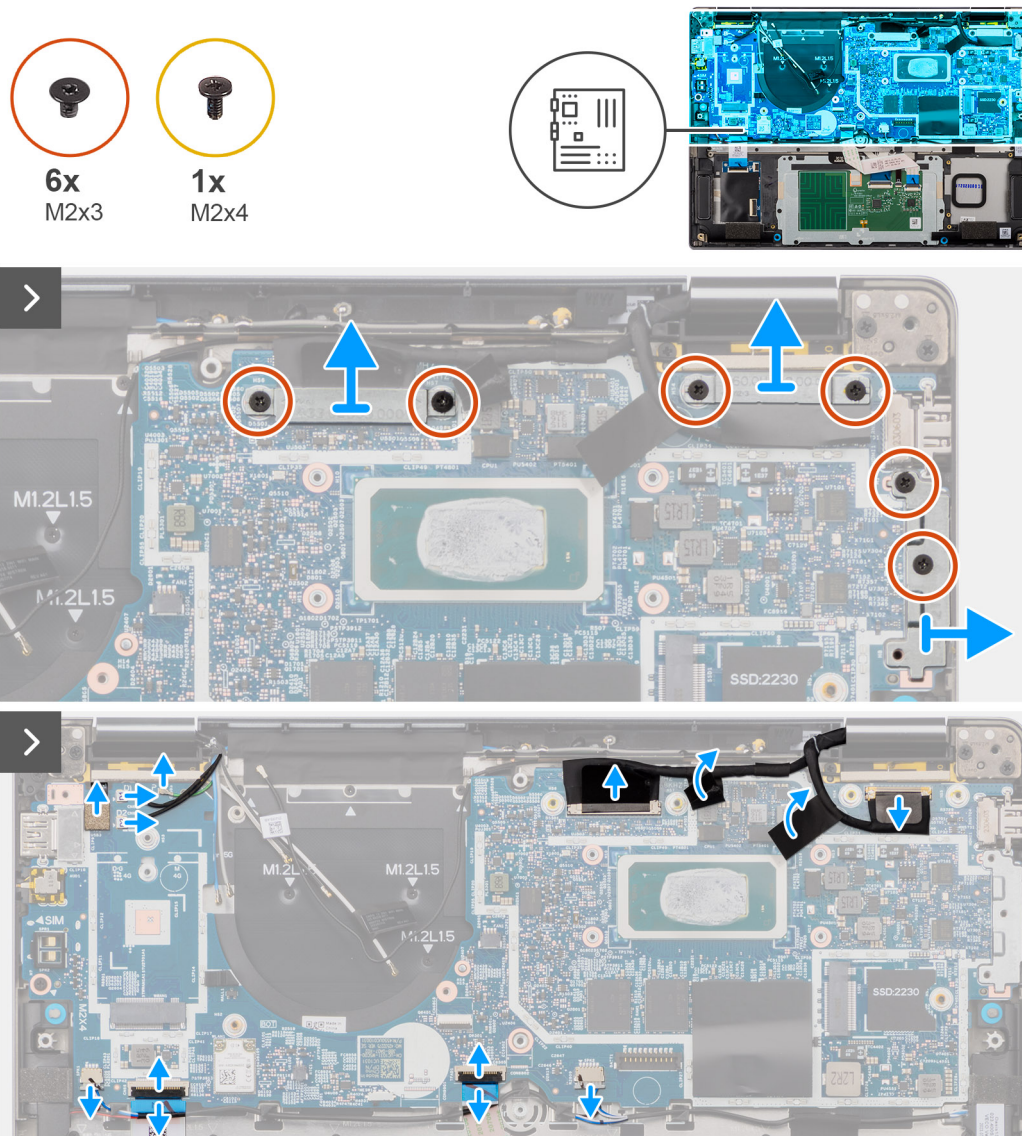
Obrázek 49. Demontáž základní desky
