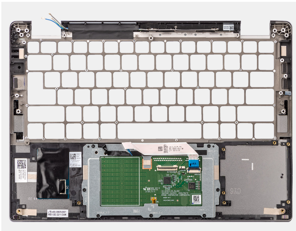
Obrázek 68. Demontáž sestavy opěrky pro dlaň
