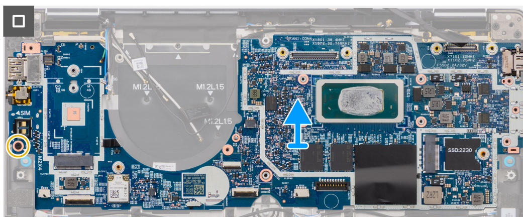
Obrázek 50. Demontáž základní desky
