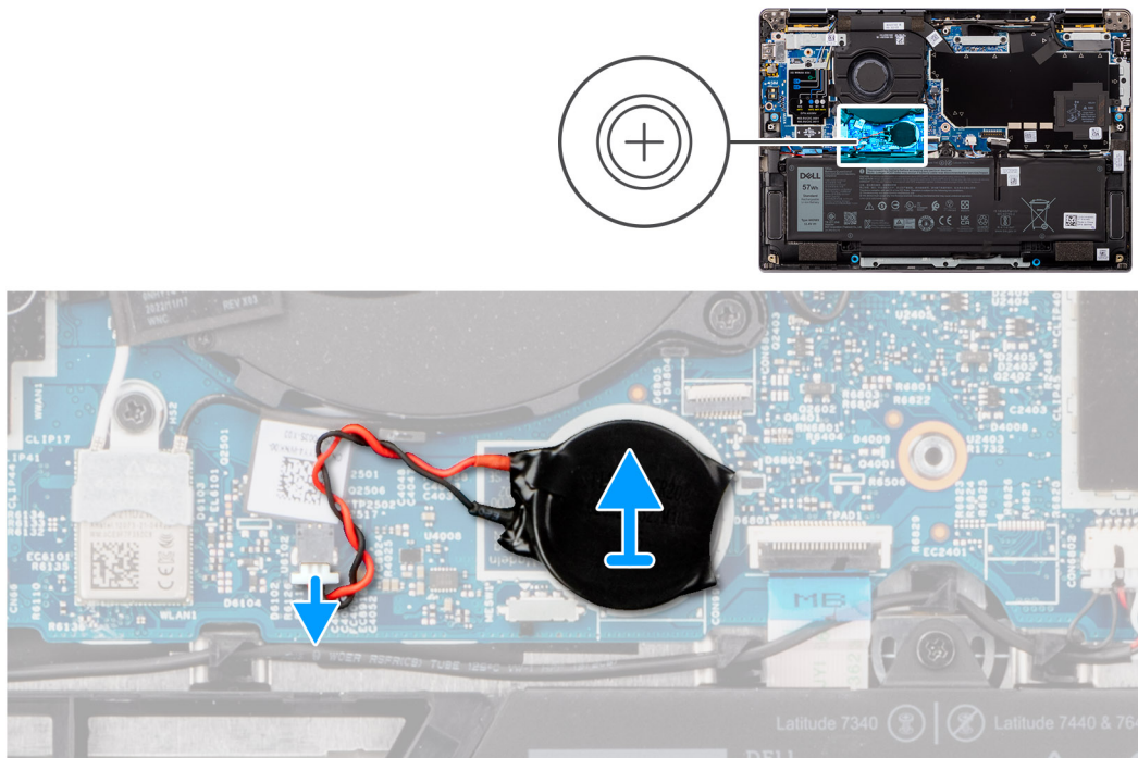
Obrázek 27. Vyjmutí knoflíkové baterie
