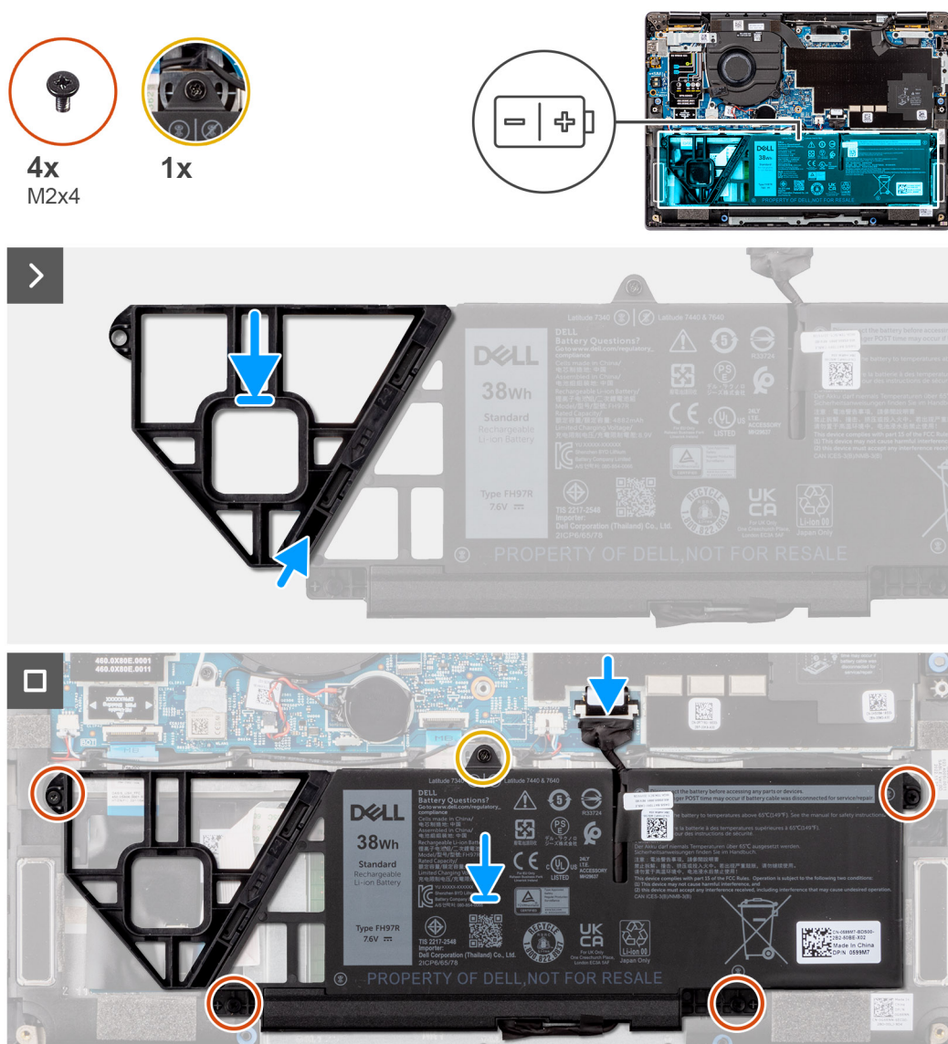
Obrázek 30. Montáž 3člankové baterie
