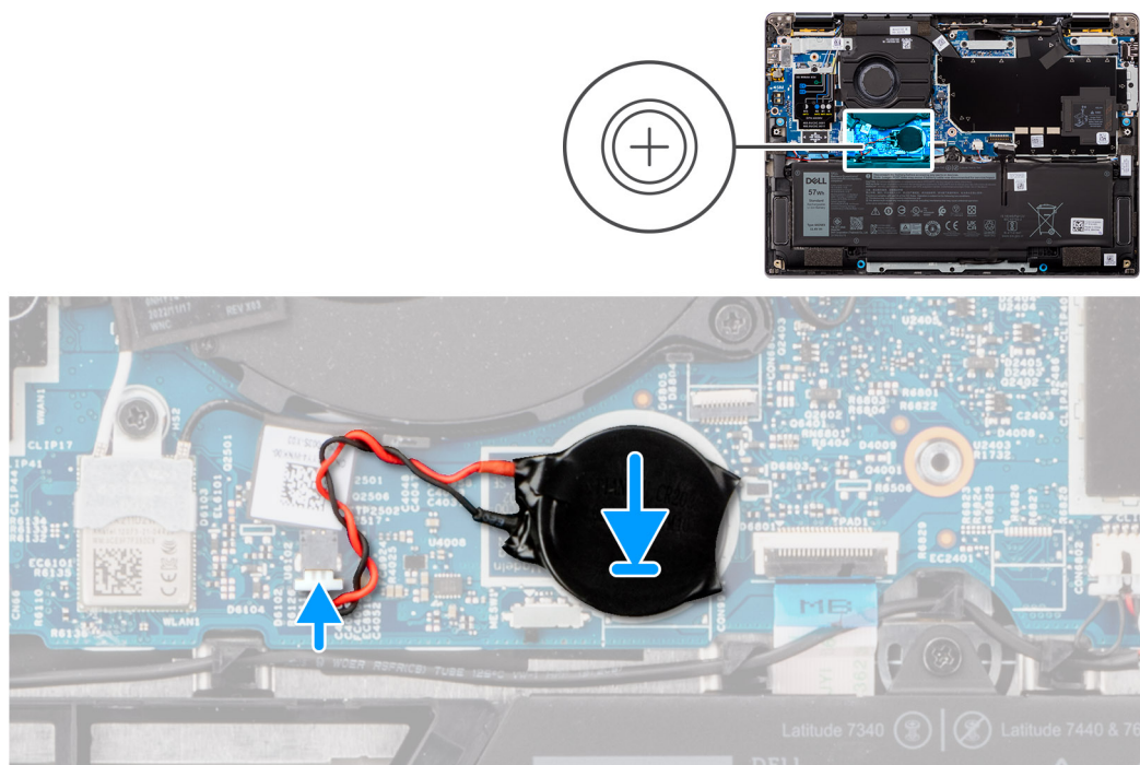
Obrázek 28. Montáž knoflíkové baterie
