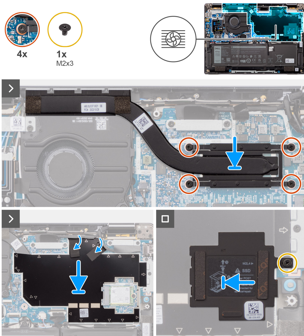
Obrázek 38. Montáž chladiče
