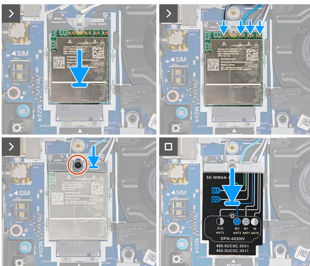
Obrázek 24. Montáž karty sítě WWAN
