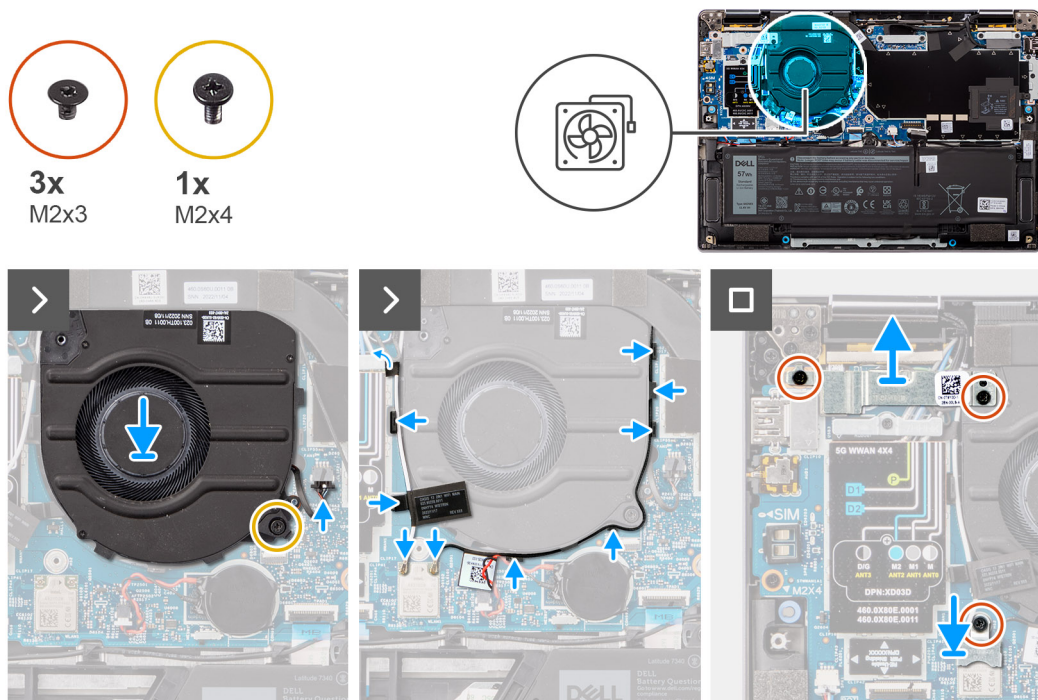
Obrázek 36. Montáž ventilátoru
