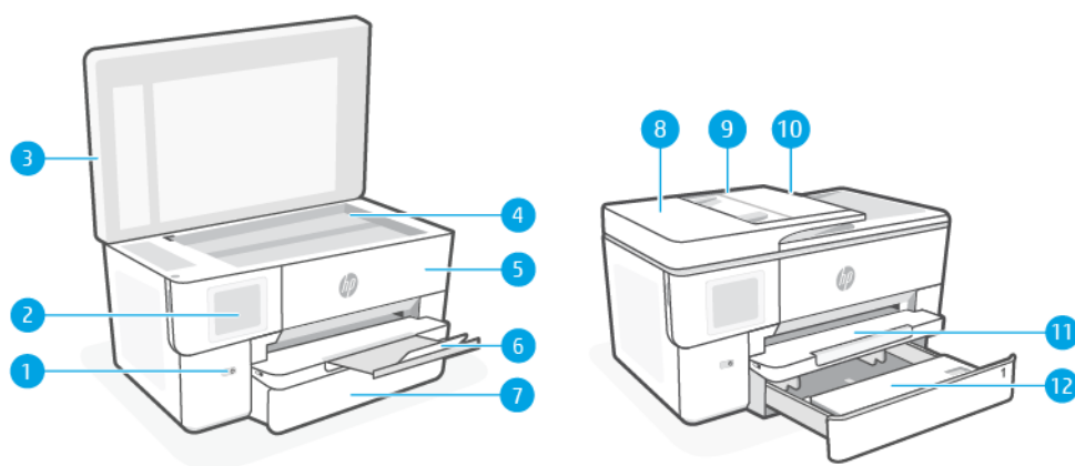
Tabulka 1-1 Pohled shora a zepředu
