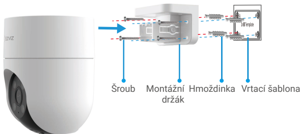
Obr. 2 Montáž na zeď
