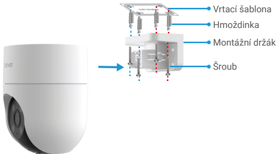
Obr. 1 Montáž na strop
