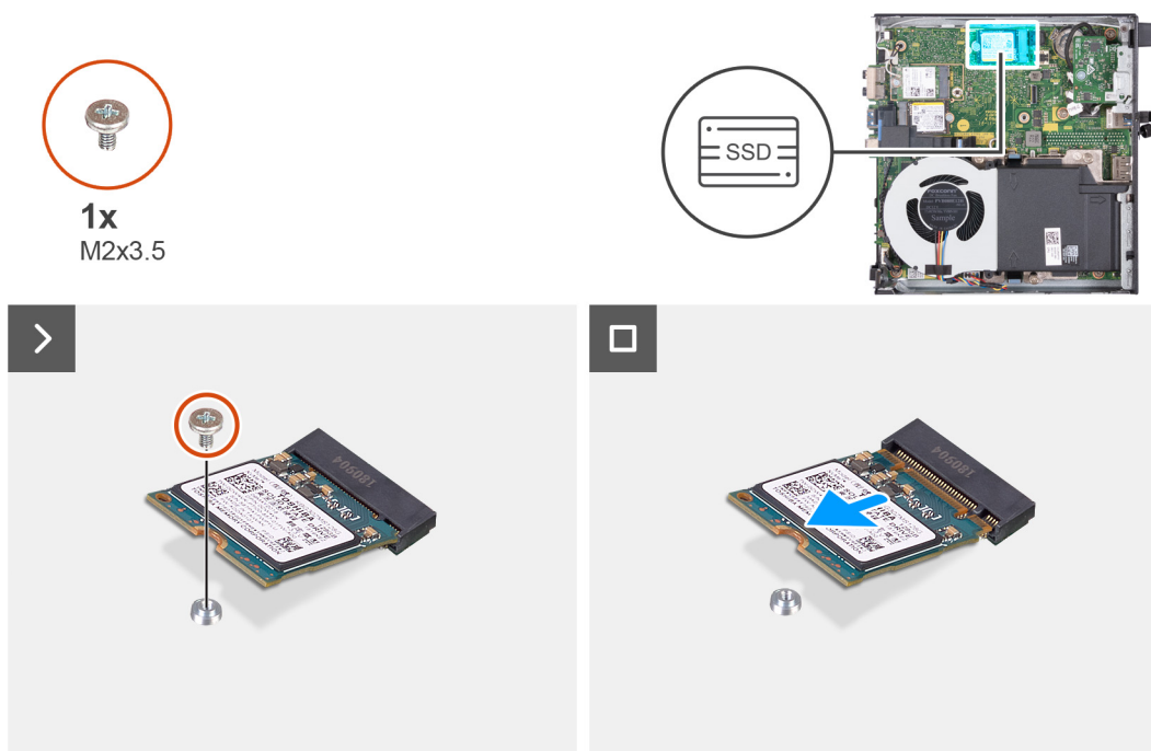
Obrázek 21. Demontáž disku SSD M.2 2230 ze slotu 1
