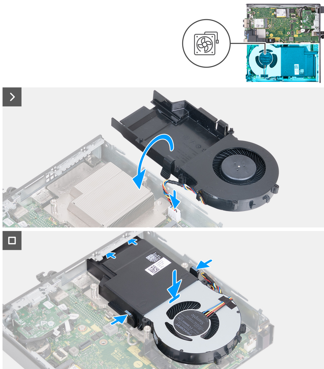
Obrázek 31. Montáž ventilátoru
