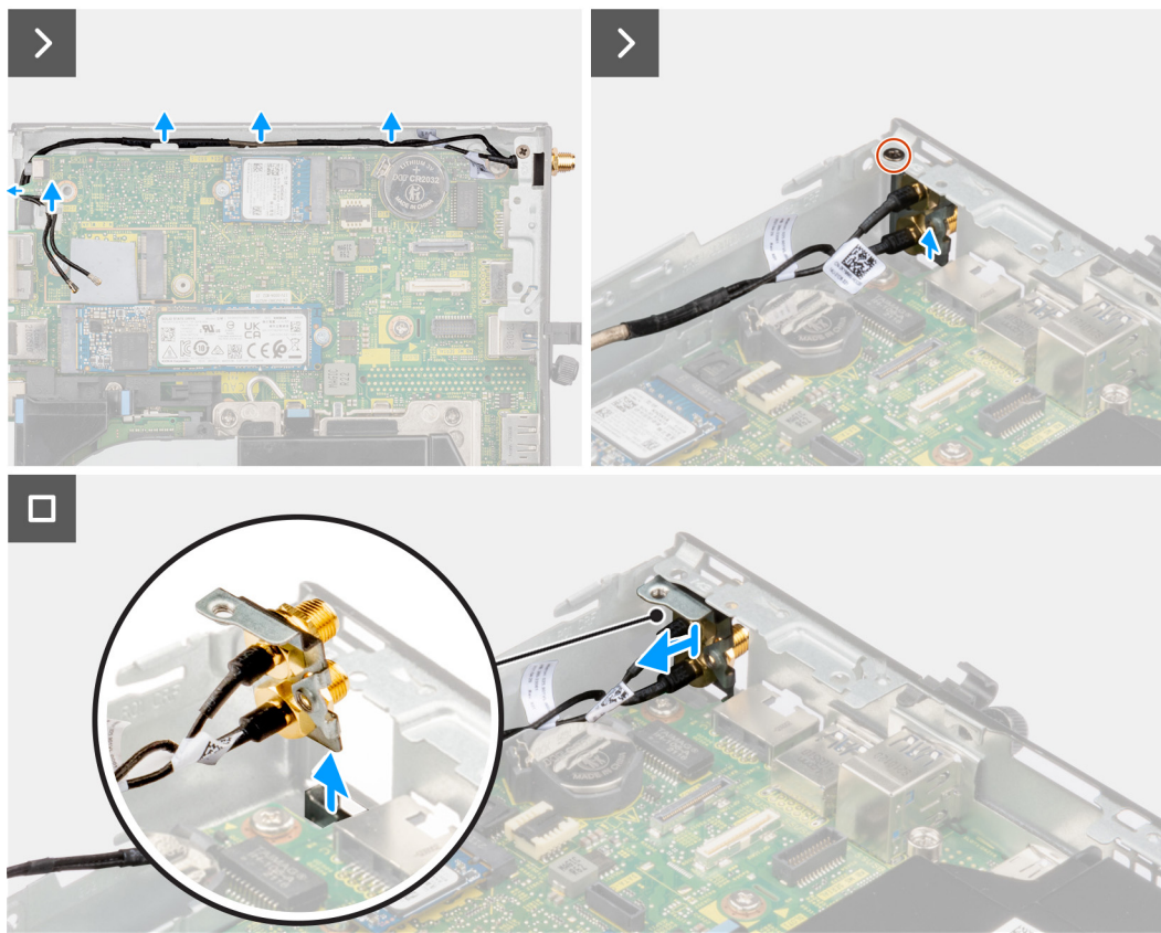
Obrázek 54. Demontáž antény SMA
