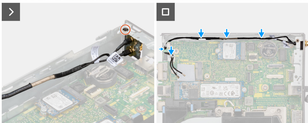
Obrázek 55. Montáž antény SMA (poloha 3)
