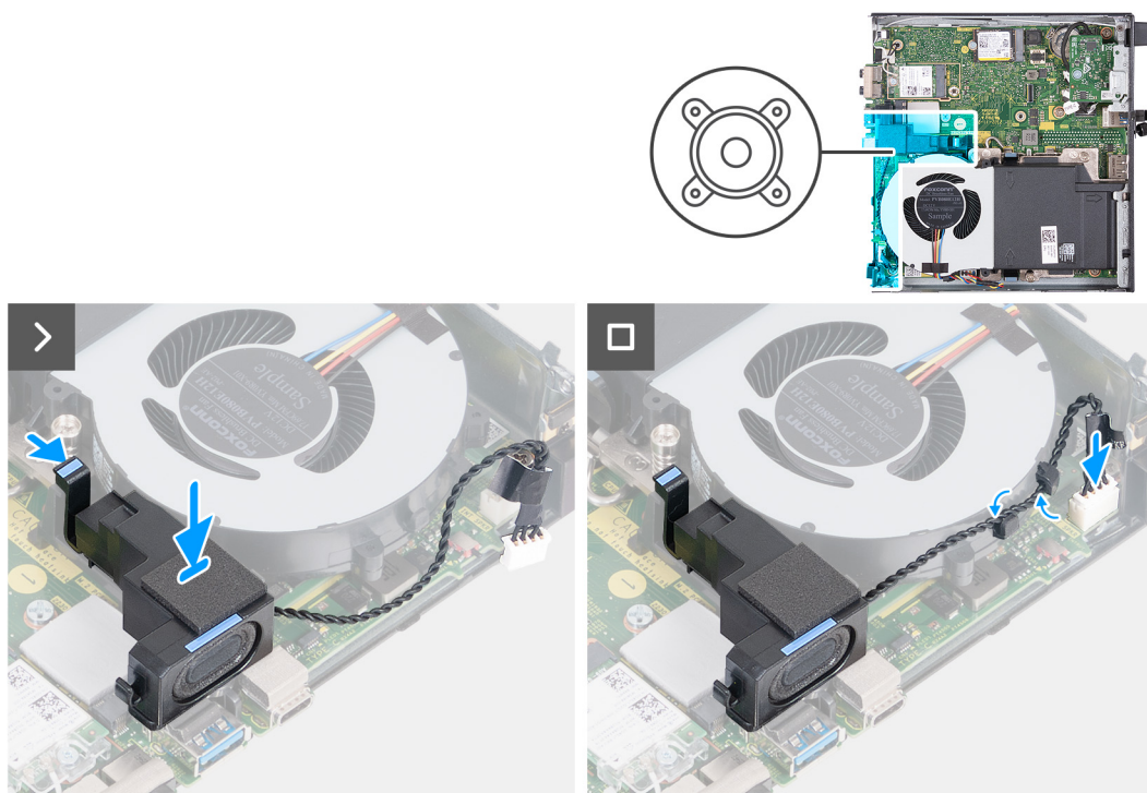
Obrázek 18. Montáž reproduktoru
