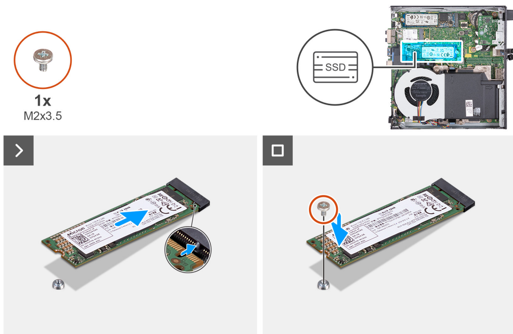
Obrázek 24. Montáž disku SSD M.2 2280 do slotu č. 0
