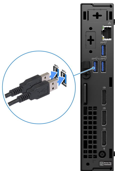
Obrázek 3. K počítači OptiPlex Micro Plus 7020 připojte klávesnici a myš.
