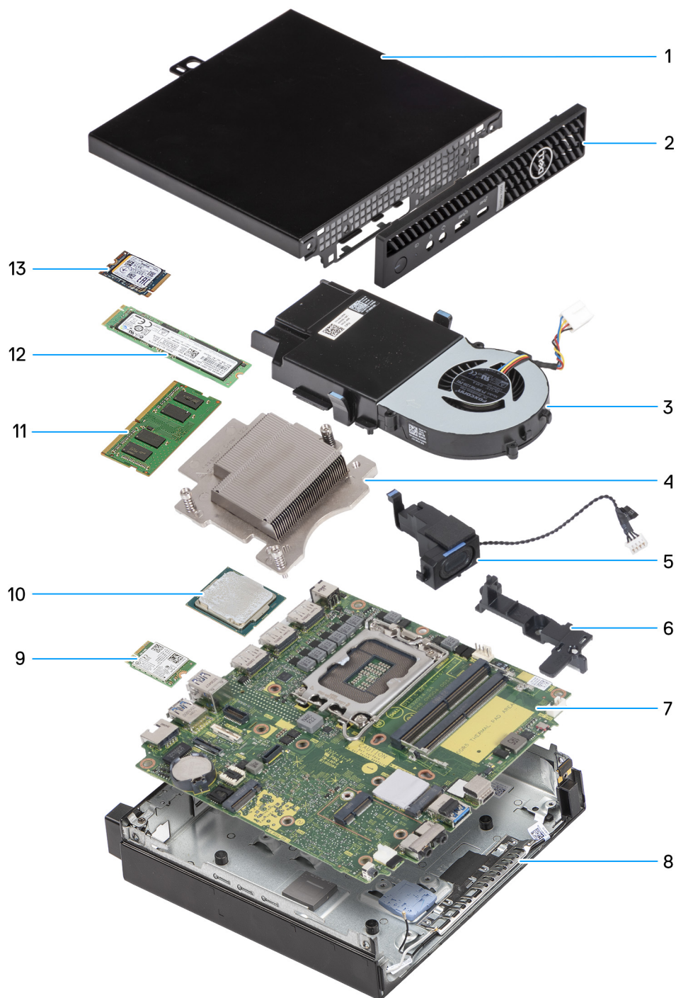
Obrázek 8. Hlavní komponenty počítače OptiPlex Micro Plus 7020
