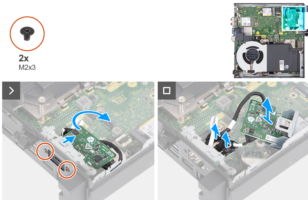
Obrázek 38. Demontáž volitelného modulu Type-C
