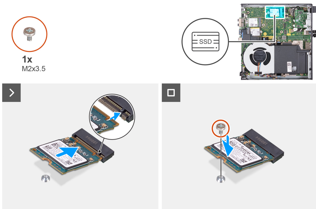
Obrázek 22. Montáž disku SSD M.2 2230 do slotu č. 1
