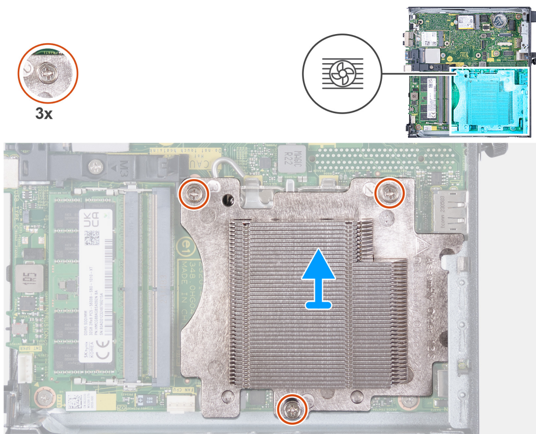
Obrázek 40. Demontáž chladiče
