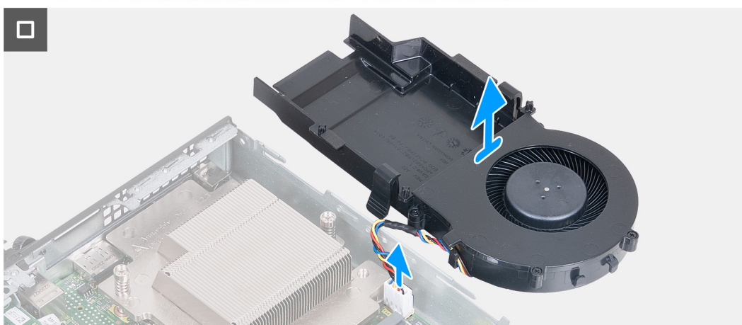
Obrázek 30. Demontáž ventilátoru
