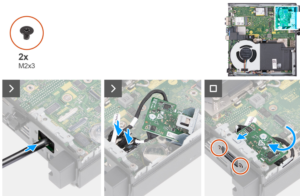
Obrázek 39. Montáž volitelného modulu Type-C
