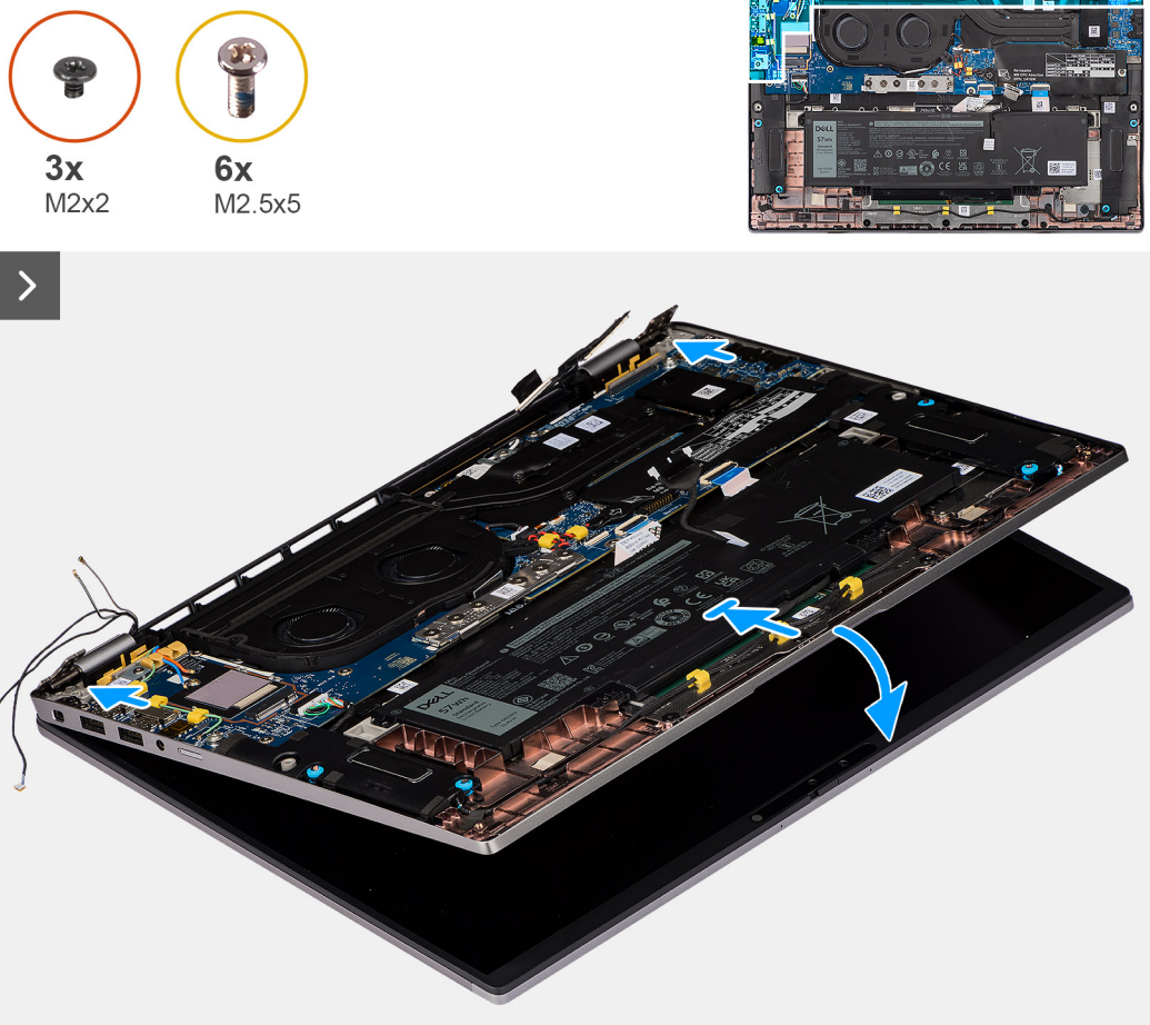
Obrázek 42. Montáž sestavy displeje
