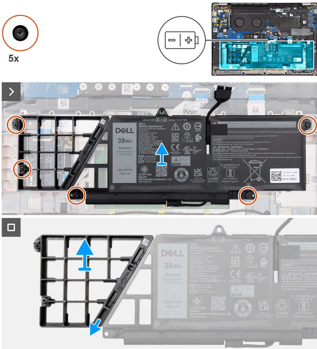
Obrázek 29. Demontáž 2článekové baterie
