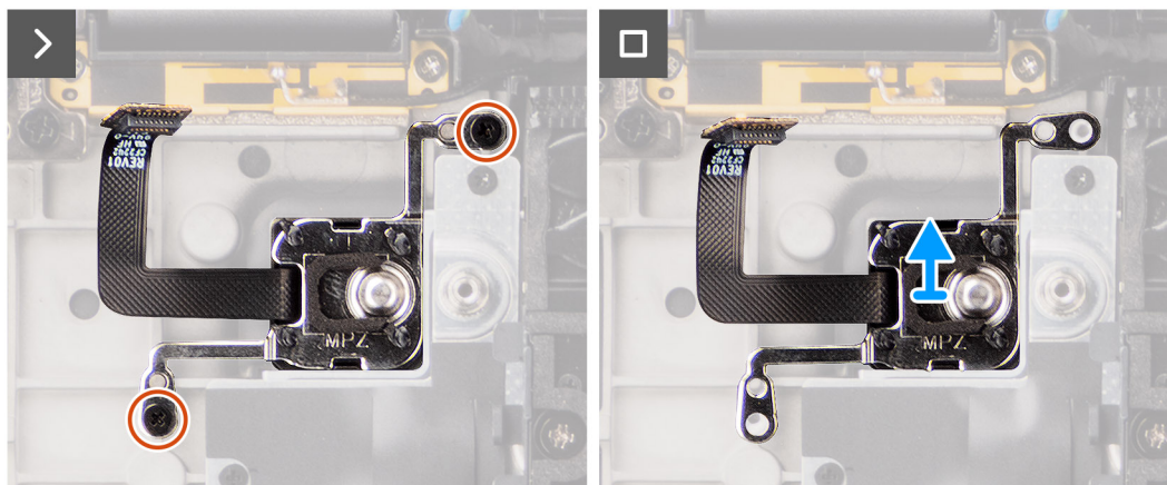
Obrázek 63. Demontáž vypínače s volitelnou čtečkou otisků prstů
