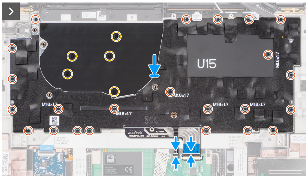
Obrázek 68. Montáž klávesnice
