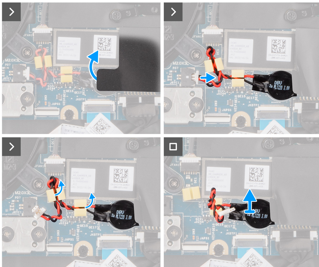
Obrázek 27. Vymutí knoflíkové baterie
