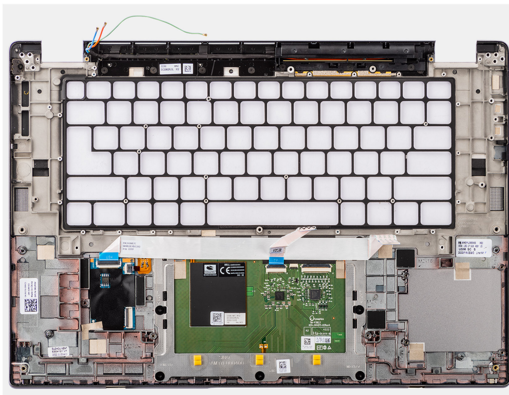
Obrázek 69. Demontáž sestavy opěrky pro dlaň
