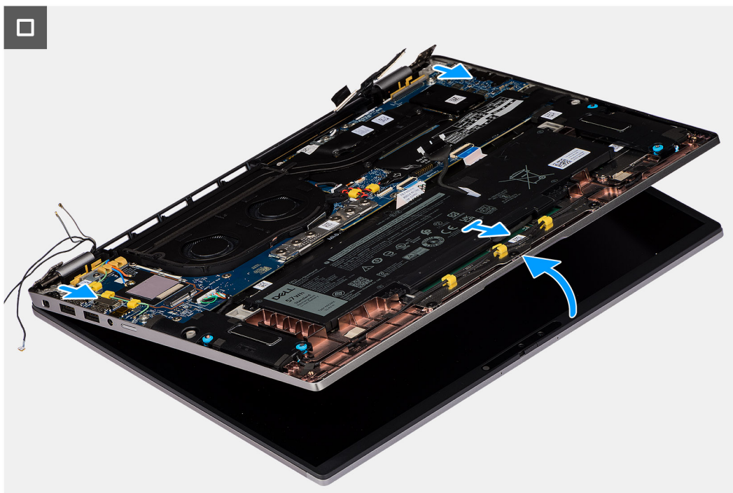
Obrázek 40. Demontáž sestavy displeje
