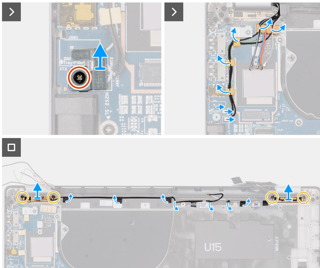
Obrázek 57. Demontáž anténního modulu WLAN
