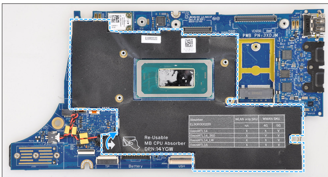
Obrázek 52. Absorbér procesoru
