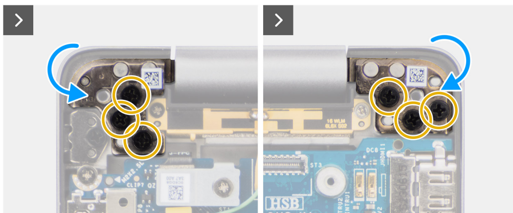
Obrázek 43. Montáž sestavy displeje
