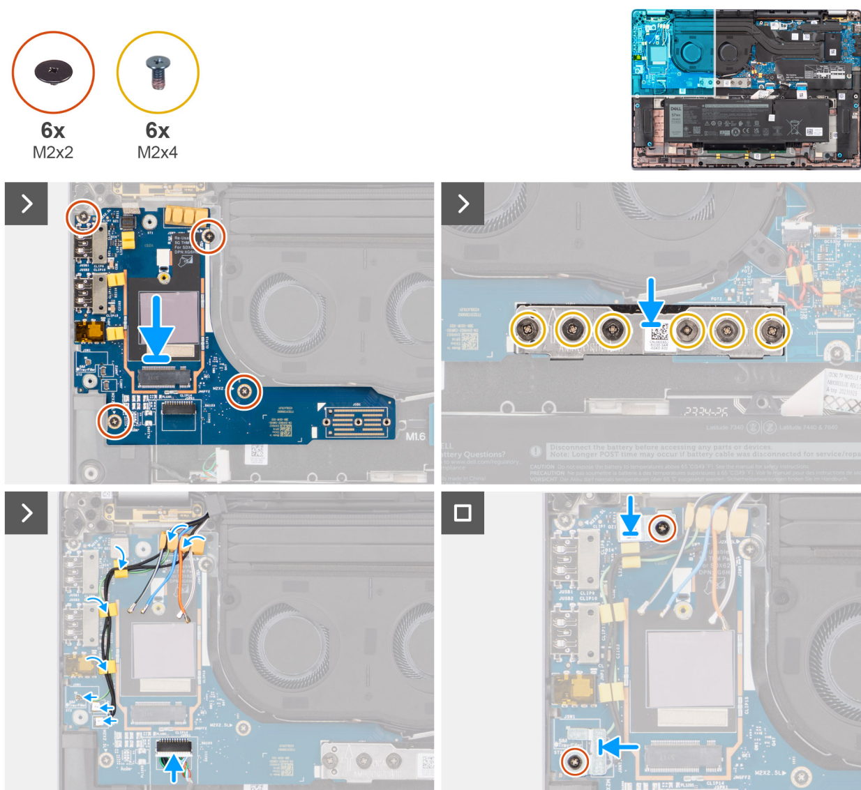
Obrázek 62. Montáž dceřiné desky I/O
