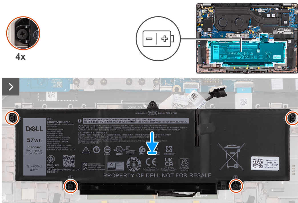
Obrázek 33. Montáž 3člankové baterie
