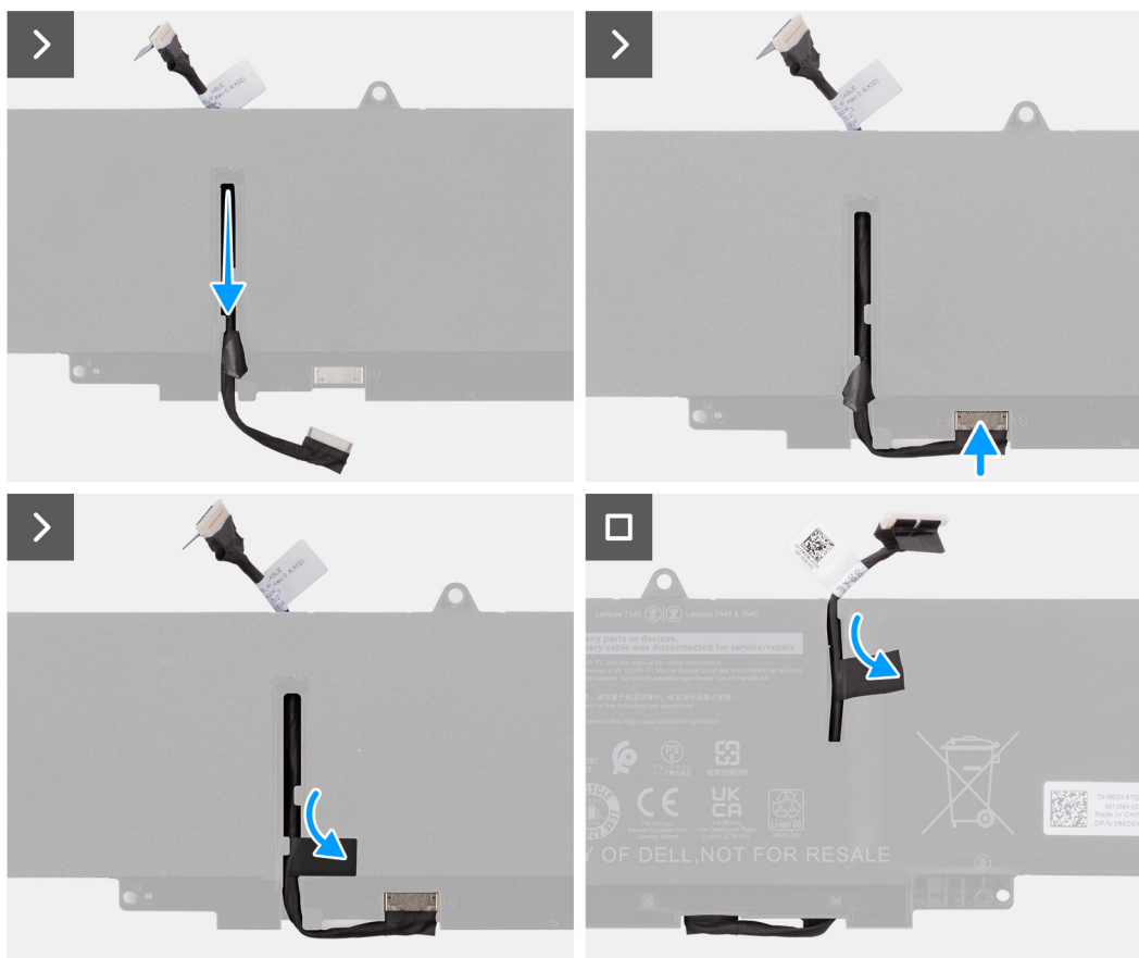
Obrázek 35. Montáž kabelu baterie
