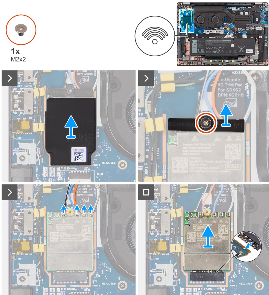
Obrázek 22. Vyjmutí karty 5G WWAN
