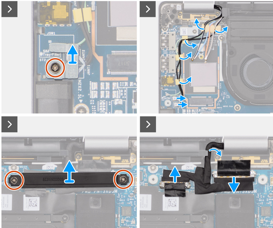
Obrázek 38. Demontáž sestavy displeje
