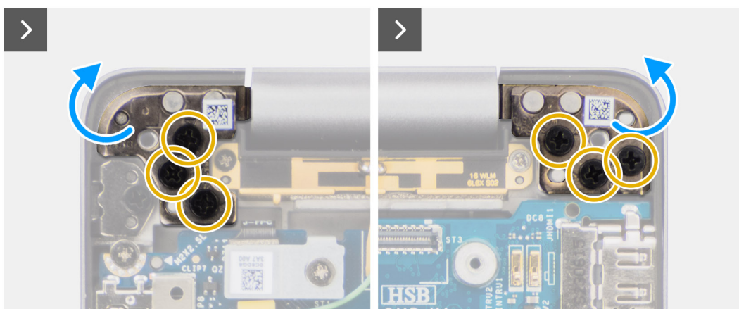
Obrázek 39. Demontáž sestavy displeje
