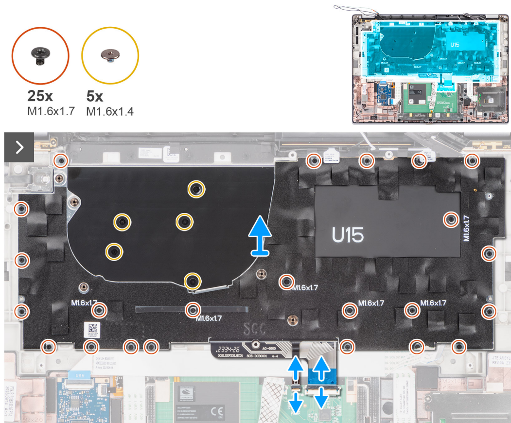
Obrázek 65. Demontáž klávesnice
