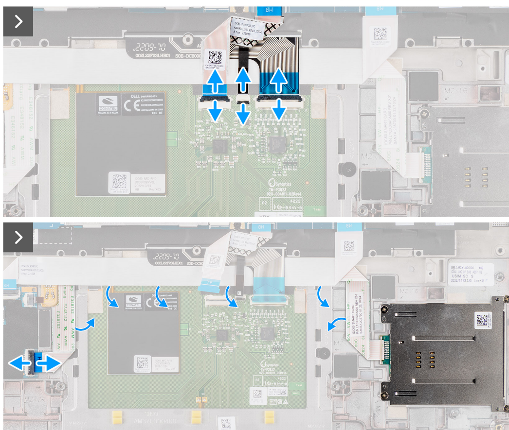
Obrázek 45. Demontáž čtečky čipových karet
