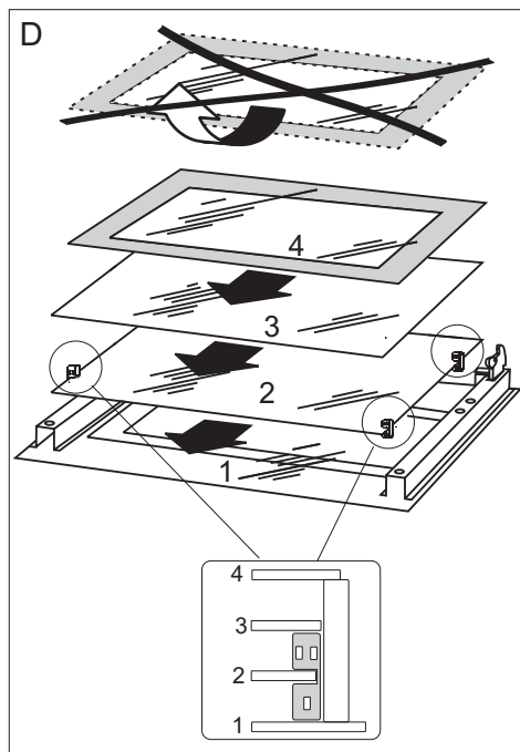
Vyjmání vnitřních skleněných tabulí
