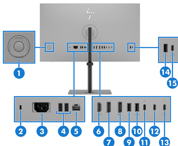
Tabulka 2-4 Součásti na zadní straně a jejich popis (modely QHD a UHD)
