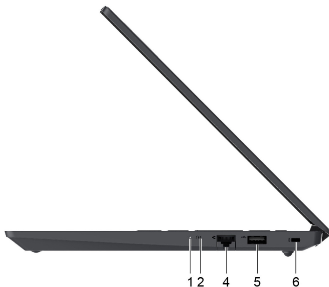
Obrázek 10. Pohled z pravé strany—Lenovo V14 G4 IRU, Lenovo V14 G4 IAH a Lenovo V14 G4 ABP
