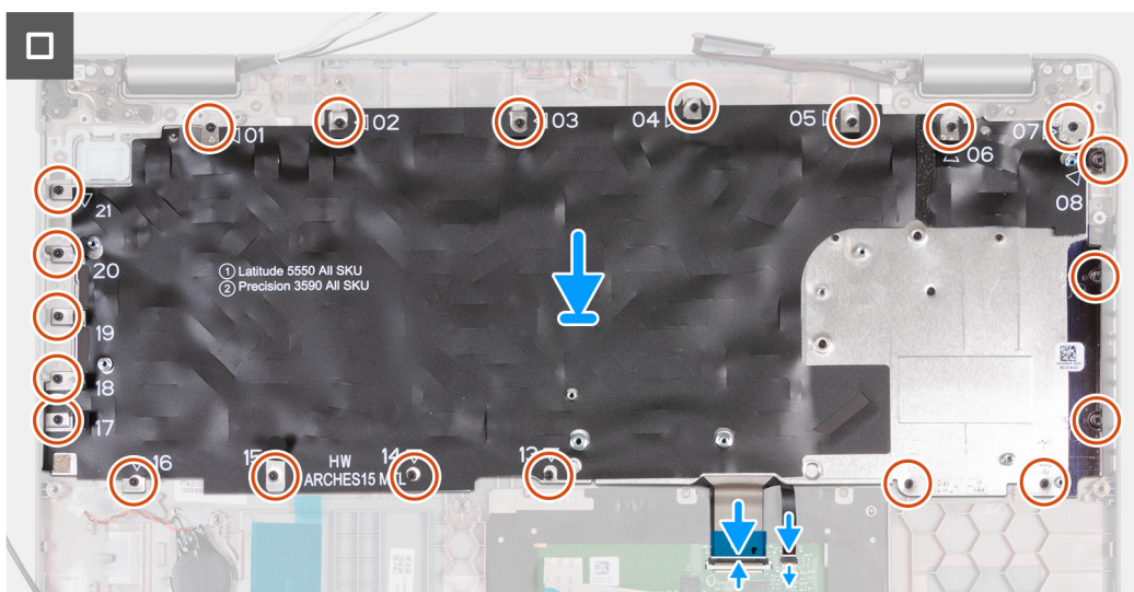
Obrázek 68. Montáž klávesnice
