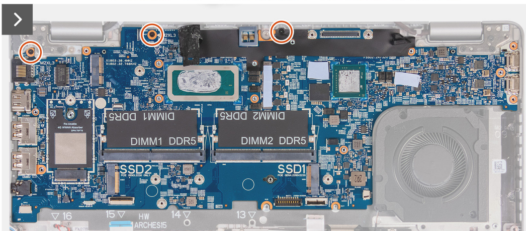
Obrázek 58. Montáž základní desky
