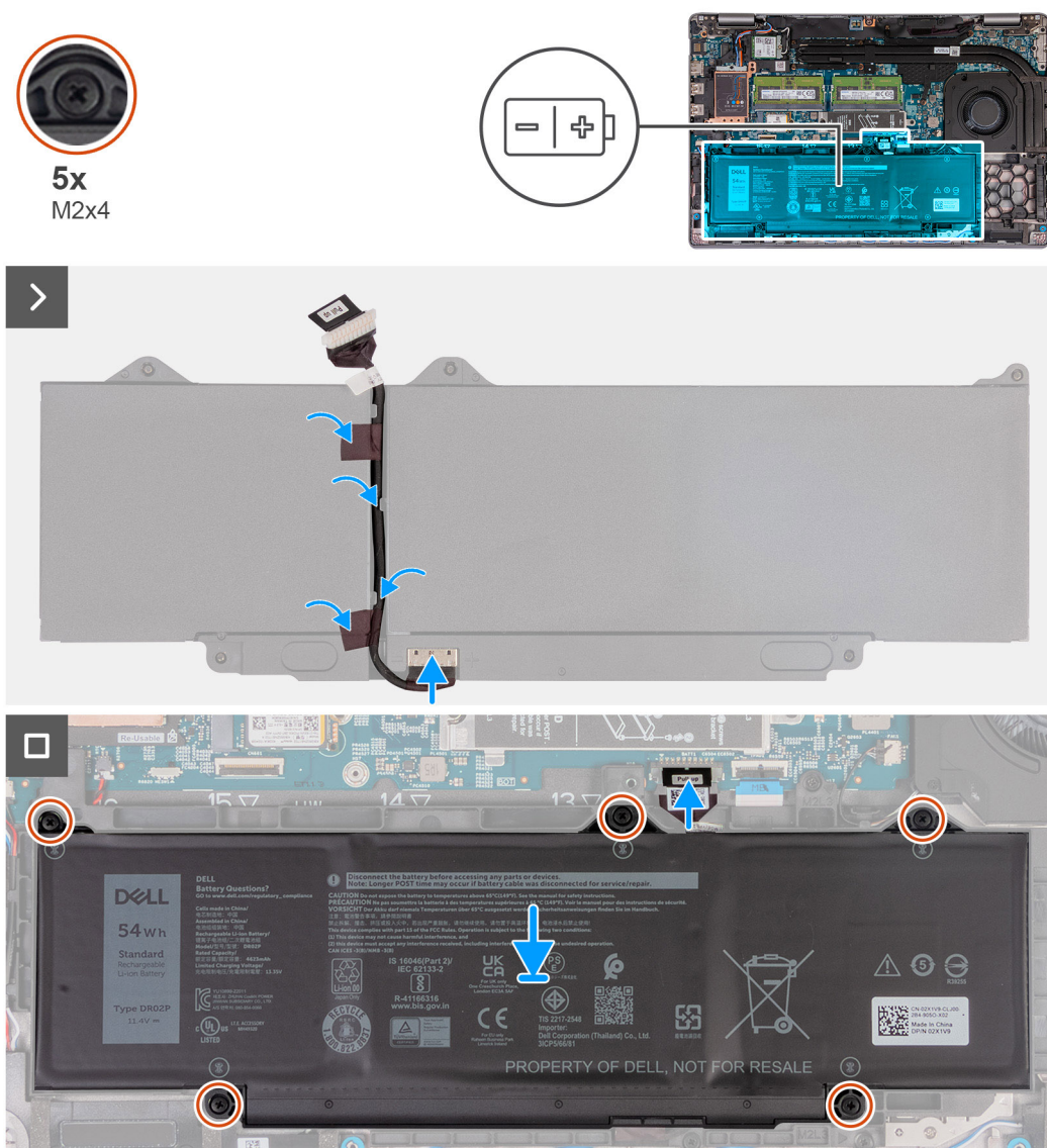
Obrázek 36. Vložení baterie
