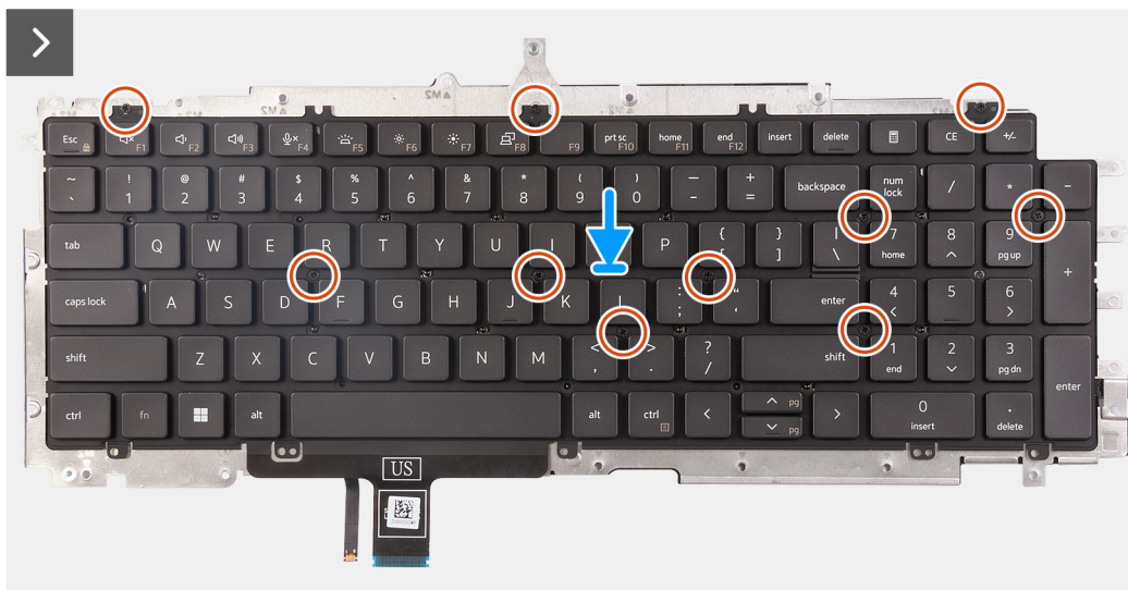
Obrázek 67. Montáž klávesnice
