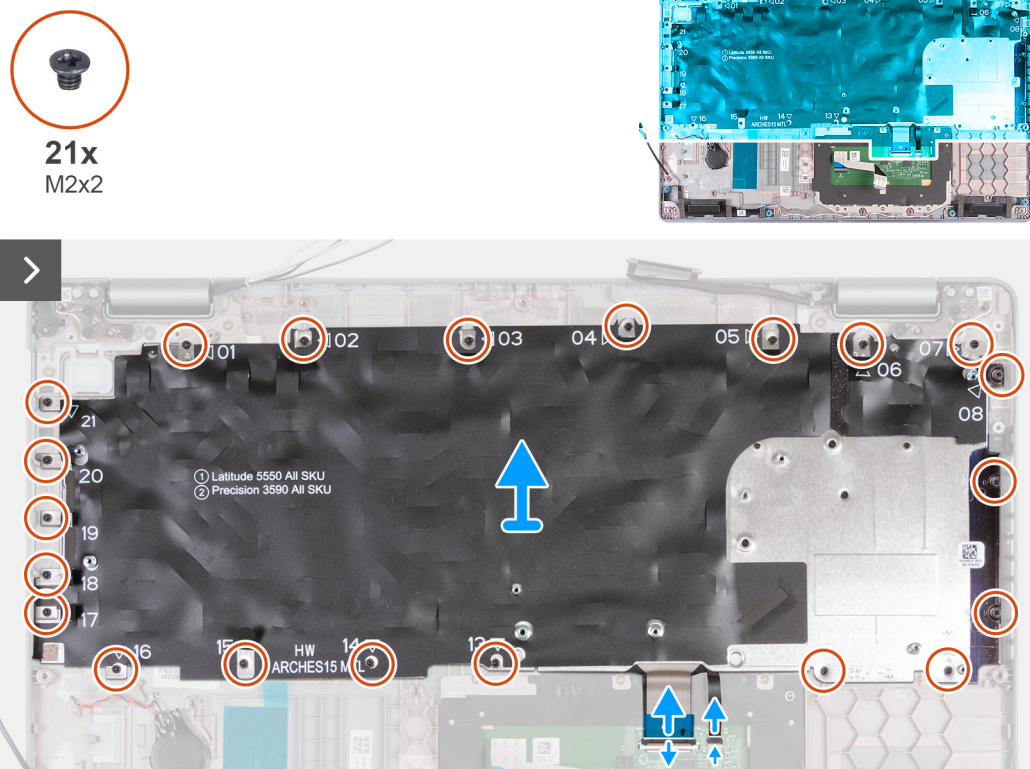
Obrázek 65. Demontáž klávesnice
