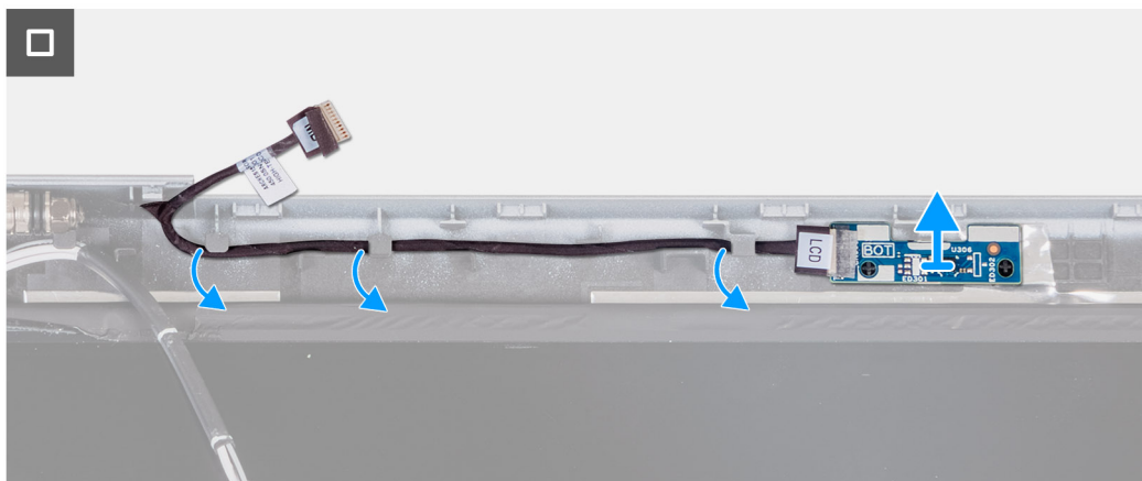
Obrázek 92. Demontáž desky snímače
