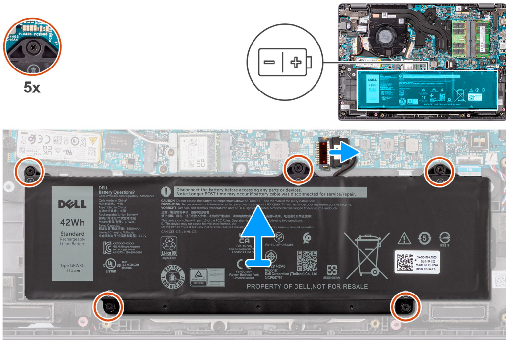
Obrázek 24. Vyjmutí baterie
