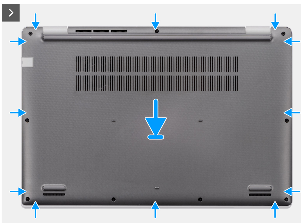
Obrázek 10. Nasazení spodního krytu
