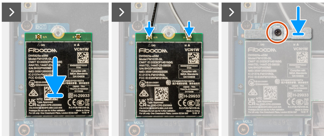
Obrázek 17. Montáž karty sítě WWAN
