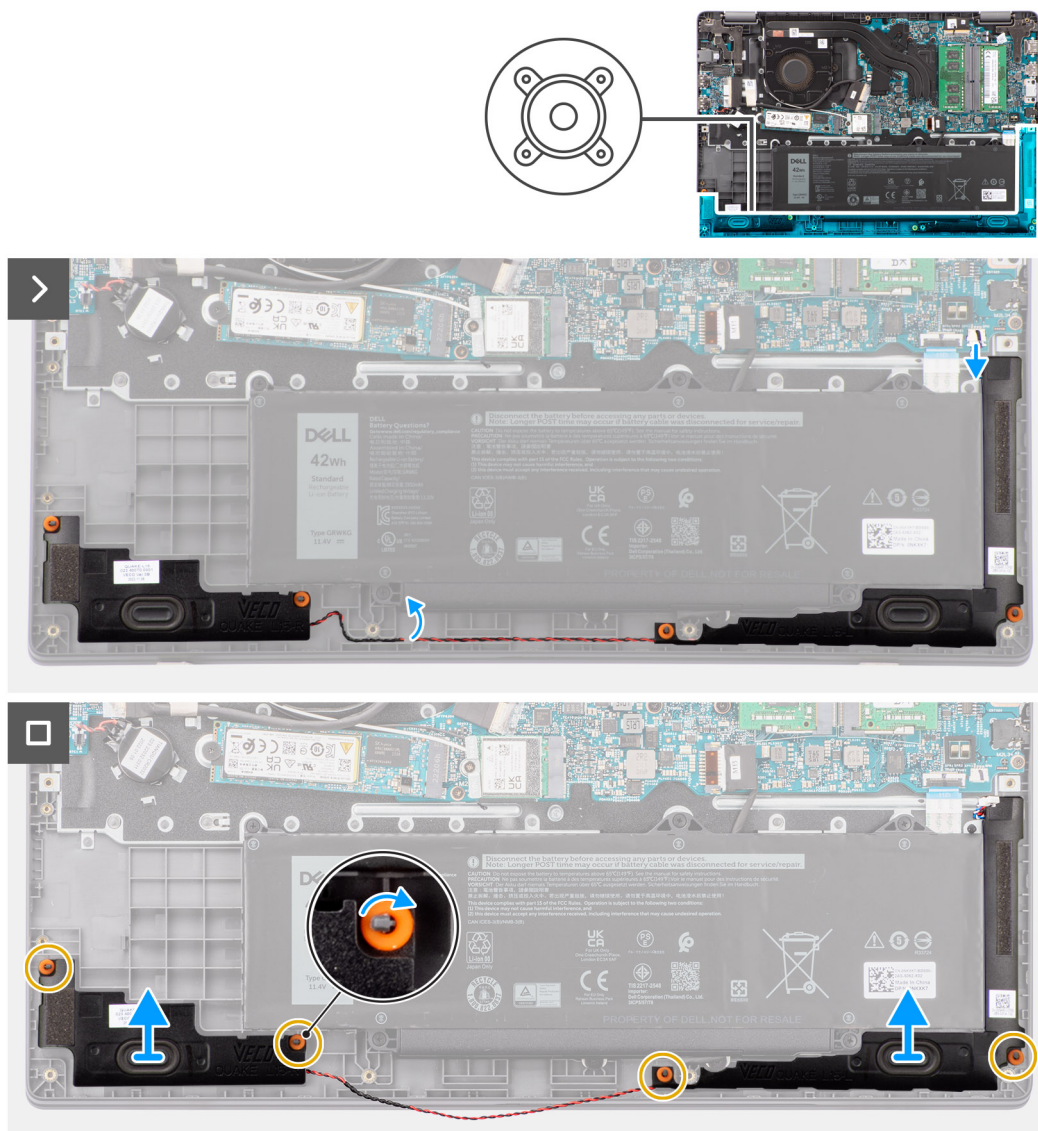
Obrázek 20. Demontáž reproduktorů
