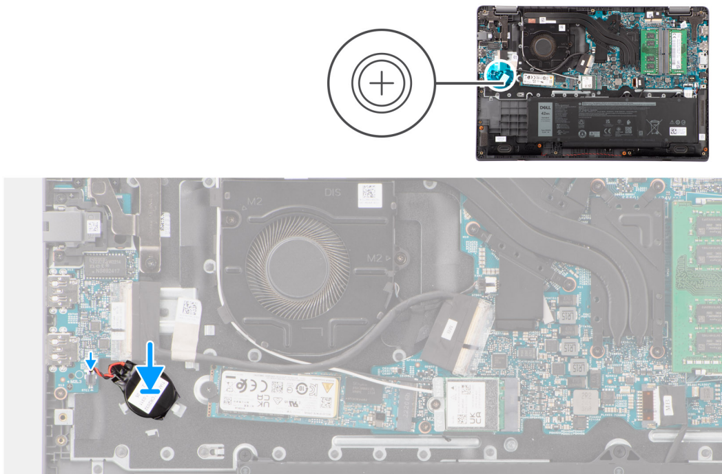
Obrázek 19. Montáž knoflíkové baterie
