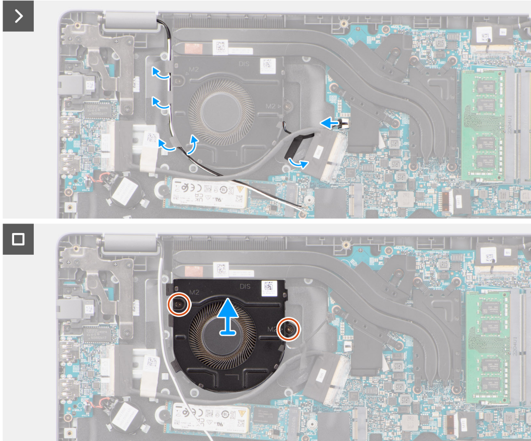
Obrázek 33. Demontáž ventilátoru
