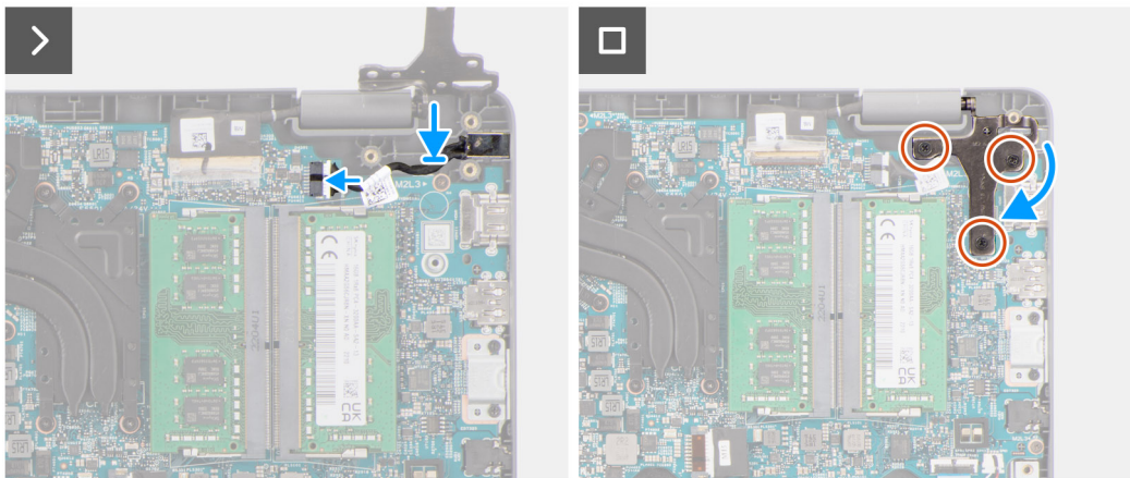
Obrázek 28. Montáž portu napájecího adaptéru
